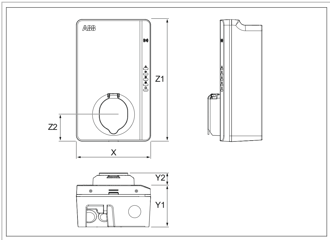
Abb. 11: Wechselstrom-Eingang mit Buchse, Kabel Typ 2
