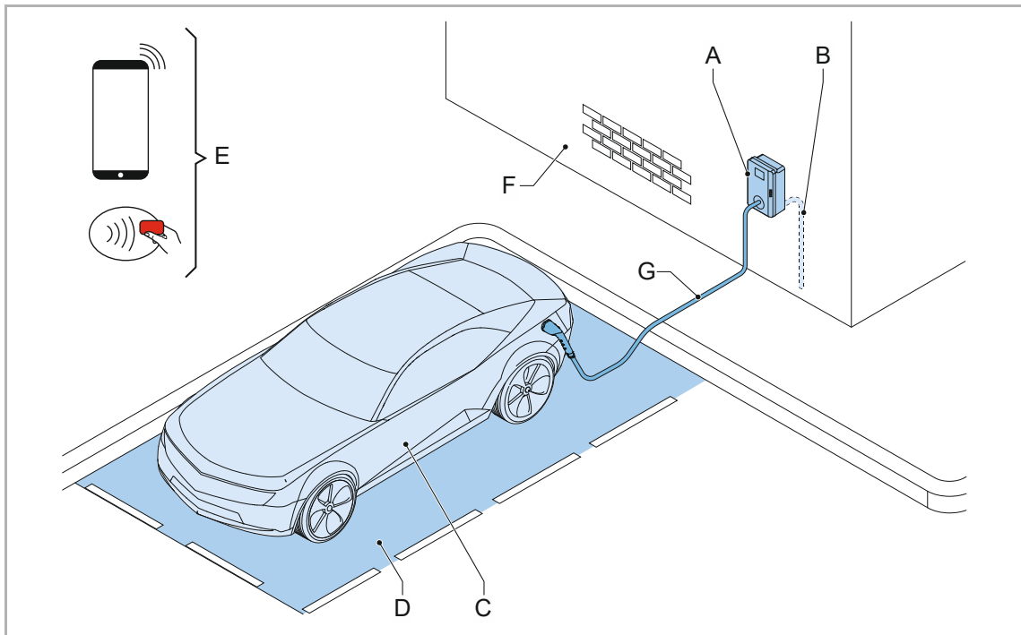
Abb. 3: Überblick über das System
