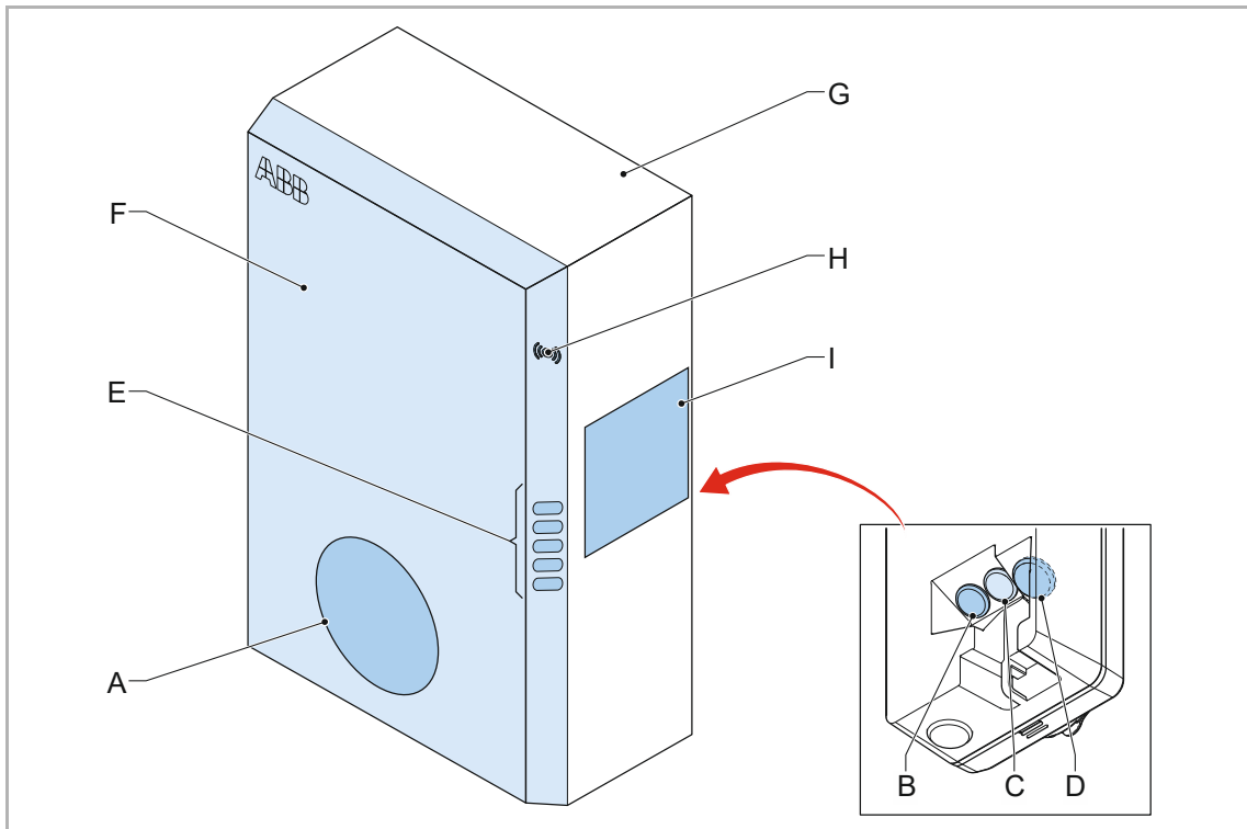
Abb. 4: Überblick über die Wandladestation - Außenansicht
