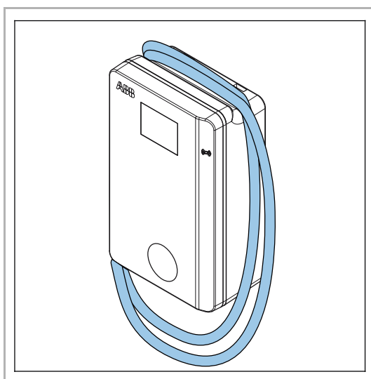
Abb. 10: Elektrofahrzeug-Ladekabel um das Gehäuse wickeln
