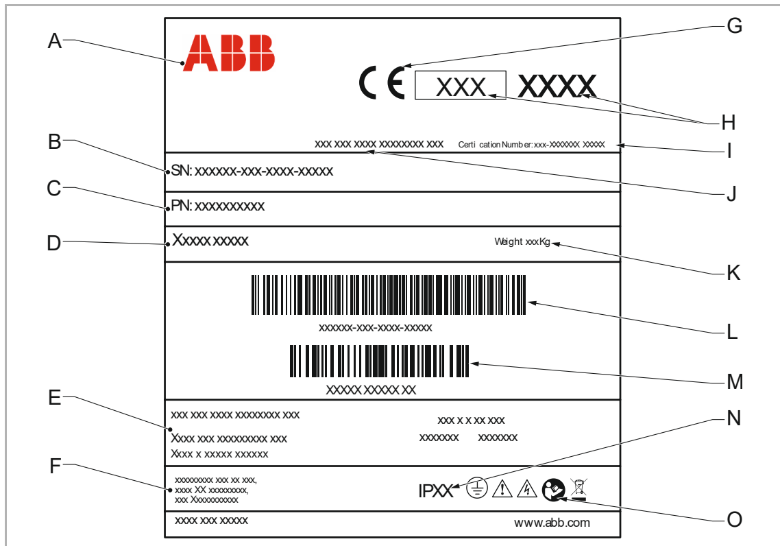
Abb. 2: Typenschild
