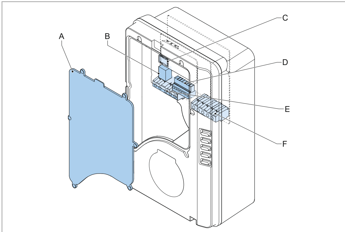
Abb. 5: Überblick über die Wandladestation - Innenansicht
